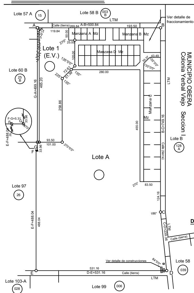
PLANO DE MENSURA ESCALA 1:5.000
